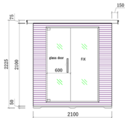
正面外観
