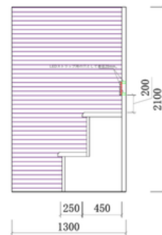
内部展開図
