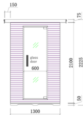
正面外観
