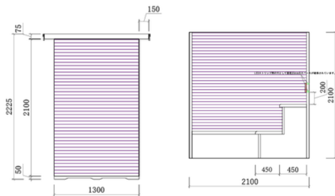
右立面図
